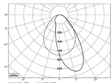
Fotometria LDT
